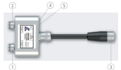
(1) KDS Tornavida #1 (2) KDS Tornavida #2 (3) KDS Kontrol Ünitesi (4) Pin GND (5) Pin IN
